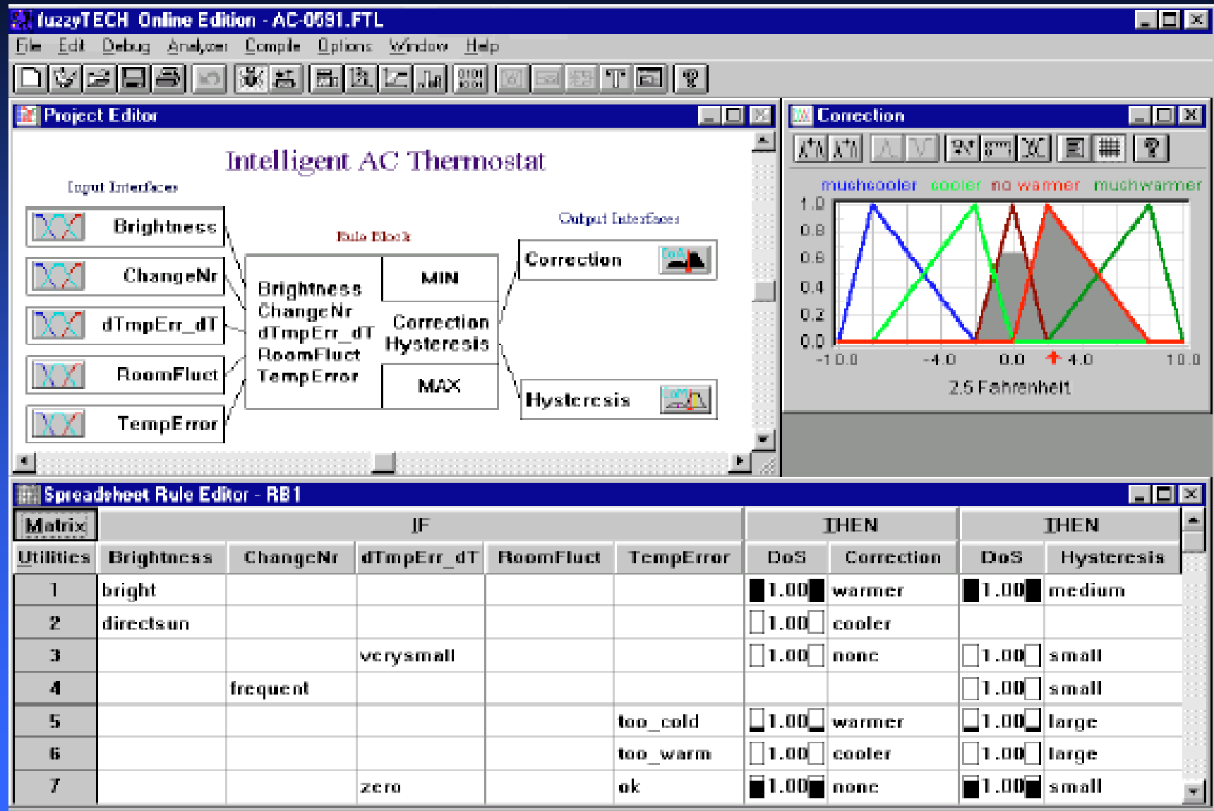
Şekil 3 : Fuzzy TECH yazılımının görünümü
