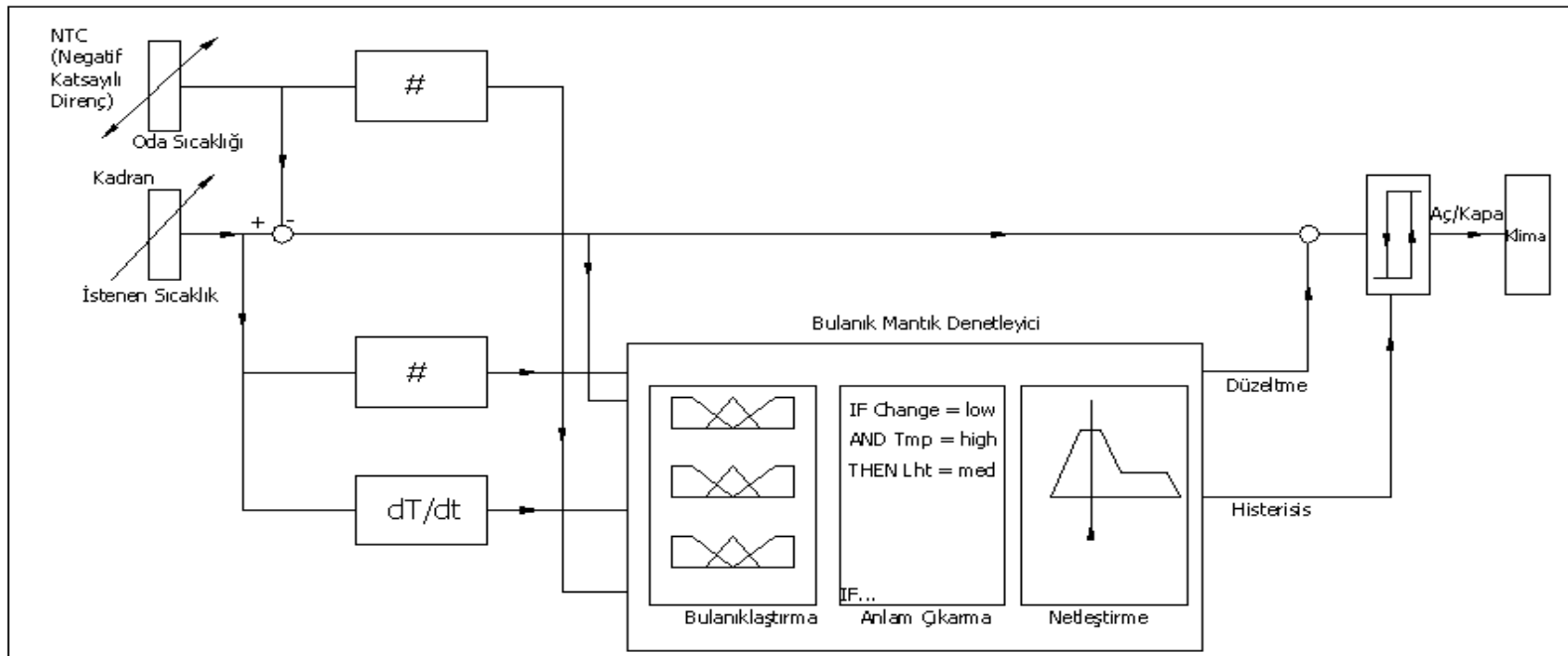
Şekil 2 : Bulanık mantık denetleyicisi hem istenen sıcaklığı hem de histerisisi odanın kullanımı ve durumuna bağlı olarak ayarlar, ki bu nedenle bulanık mantık mikro denetleyiciler de deneysel bilgilerin gerçekleştirilmesi için seçilmiştir.
