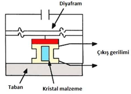
Şekil 8. Piezoelektrik basınç sensörü
