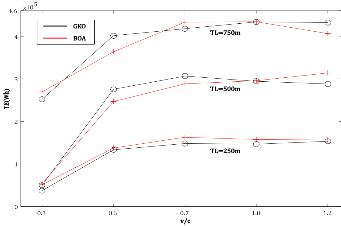
Şekil 2. GKA ve BOA'nın önerdikleri KPT planlarına ait toplam enerji transfer miktarı.
