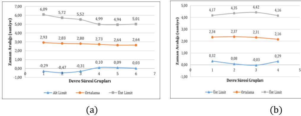
Şekil 3. Kipa (a) ve CNR (b) Kavşakları devre süresi gruplarına göre sapan değer analizi.
