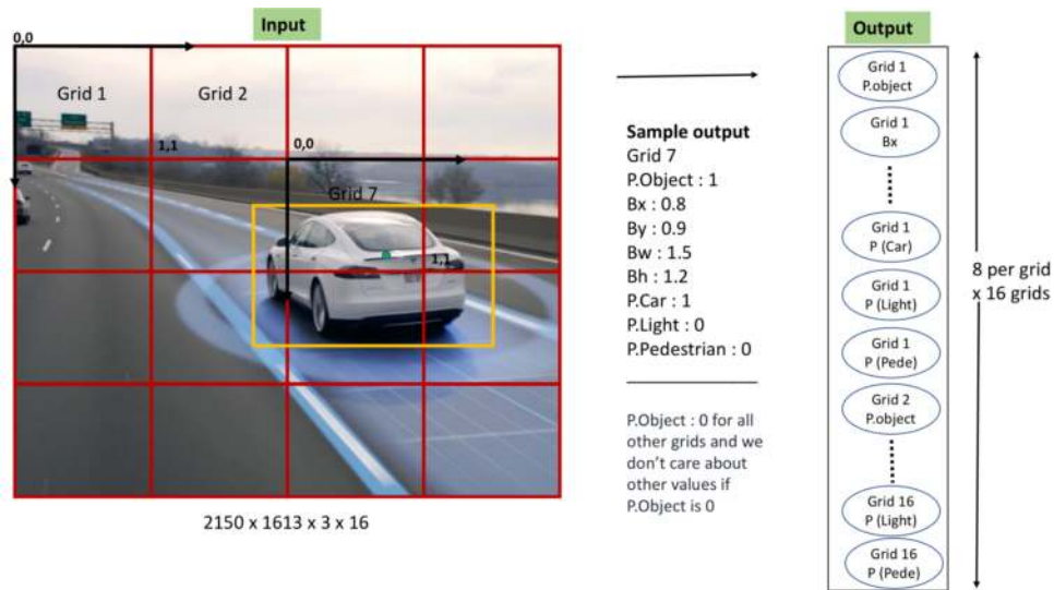
Şekil 9. YOLO algoritması çıktısı
