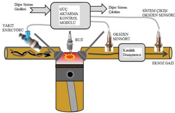
Şekil 2. Motor yanma işlemi [19]
