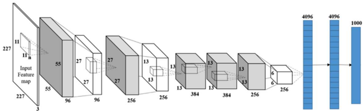
Şekil 7. YOLO algoritmasının mimari yapısı
