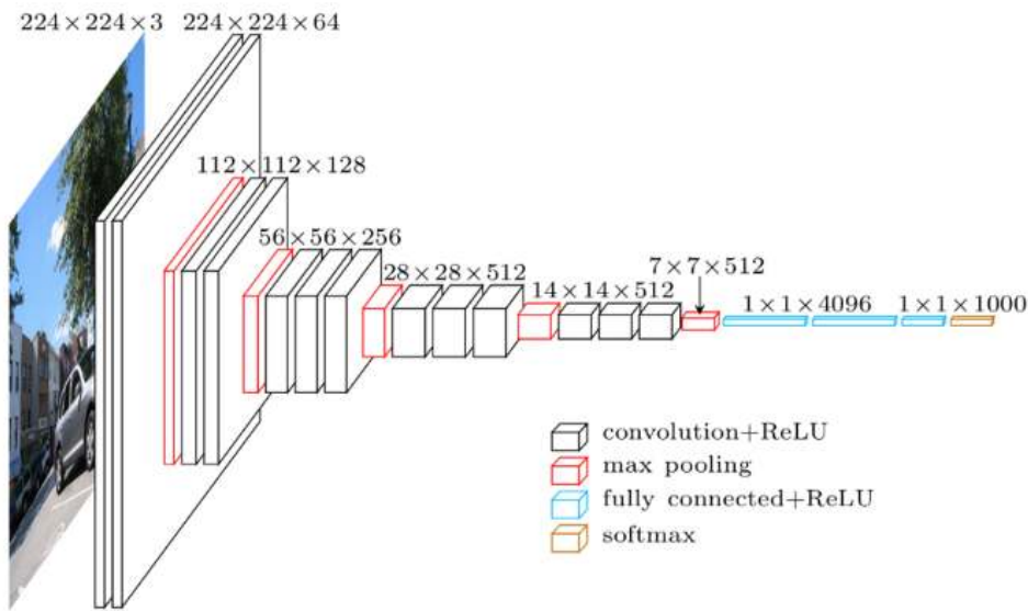
Şekil 8. ESA algoritmasının mimari yapısı
