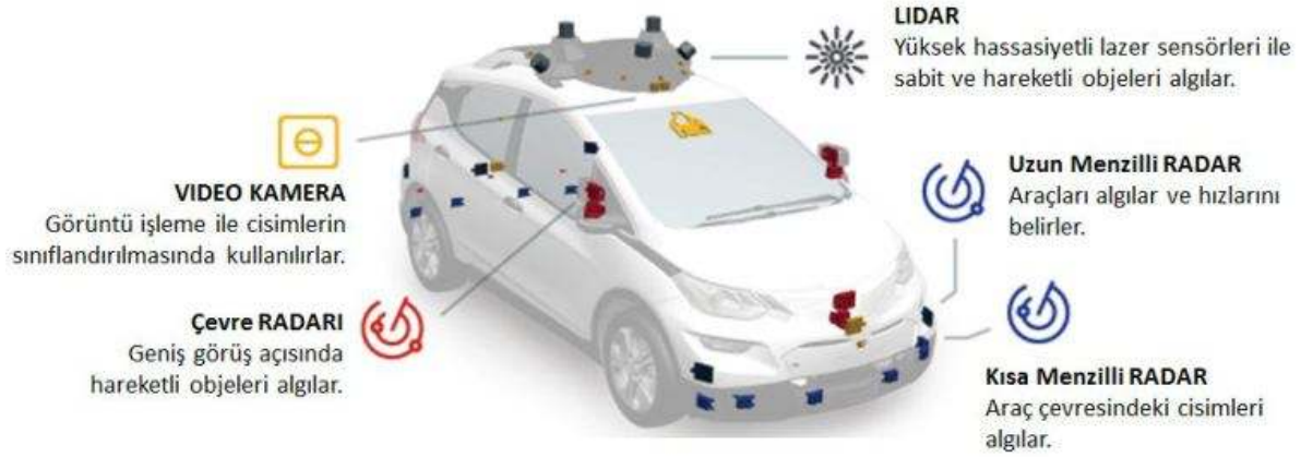
Şekil 6. Otonom Araçlarda kullanılan sensörler
