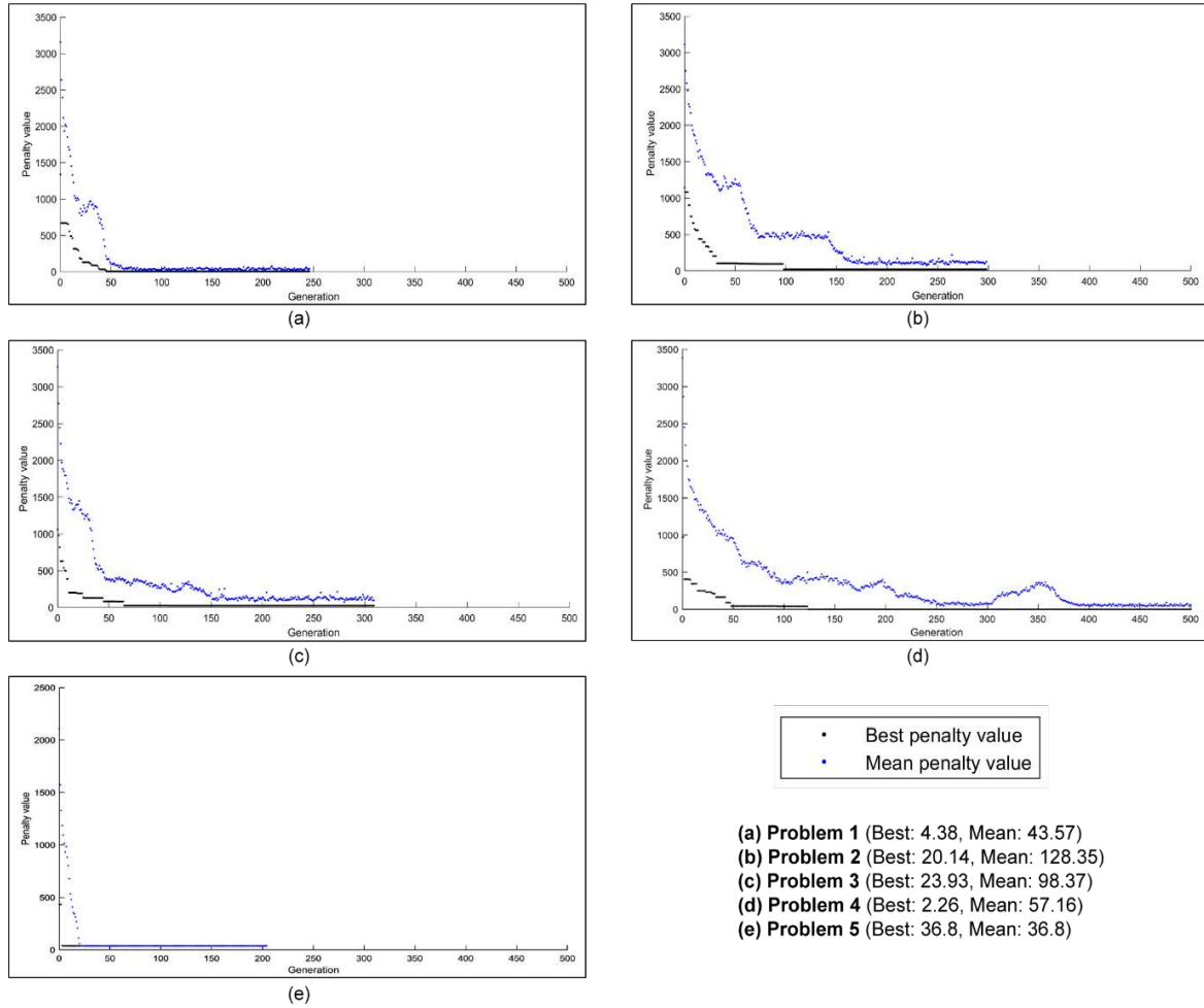
Şekil 4. GA'nın Uygunluk Fonksiyonuna Göre Ceza Değerleri
