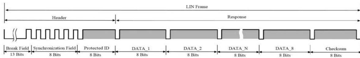
Figure 11. Frame of LIN (Zeng et al, 2016).
