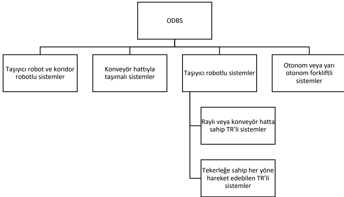
Şekil 4. ODBS türleri
