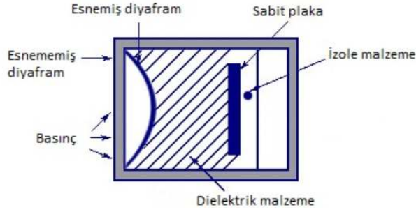
Şekil 7. Kapasitif sensör
