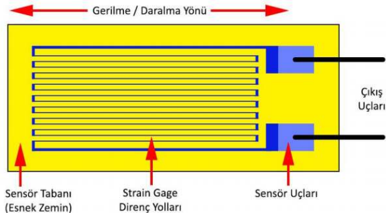
Şekil 9. Gerinim ölçer basınç sensörü
