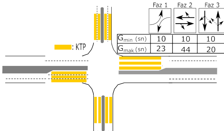
Şekil 1. Kavşak geometrisi ve sinyal kontrol sistemi özellikleri.
