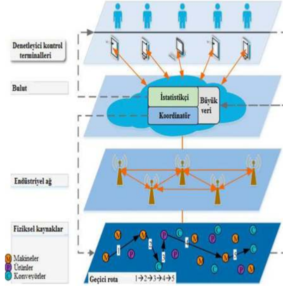
Şek.4. Akıllı Fabrika Çerçevesi [5]
