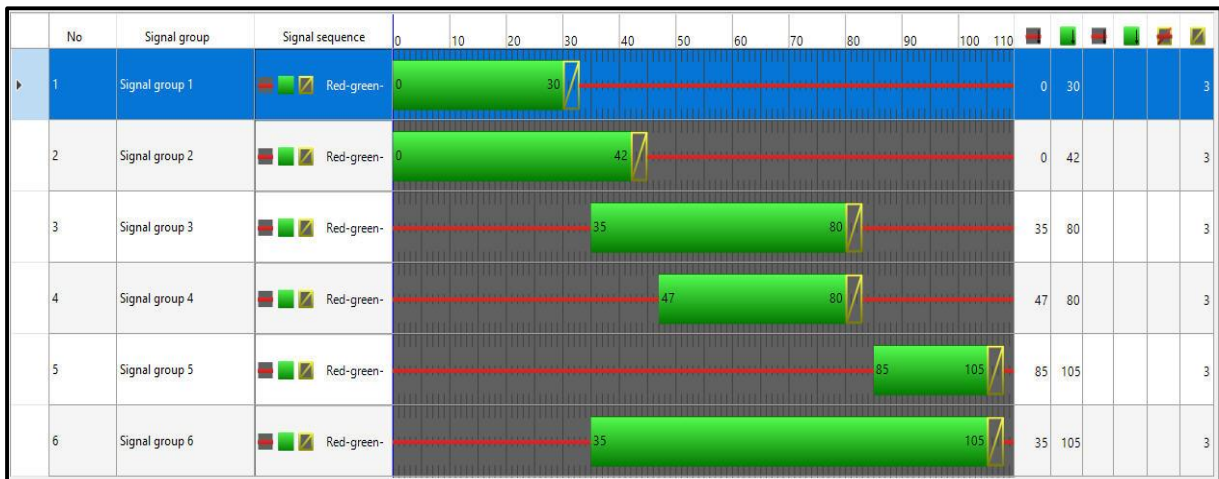
Şekil 5.9 : Revize Sinyal Planı (Akşam)
