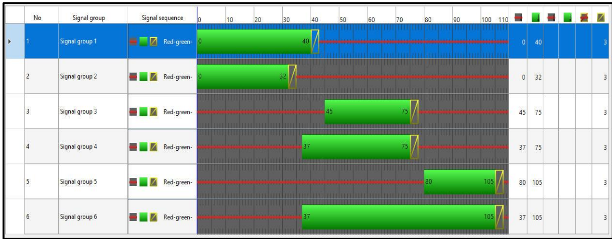
Şekil 5.8 : Revize Sinyal Planı (Sabah)
