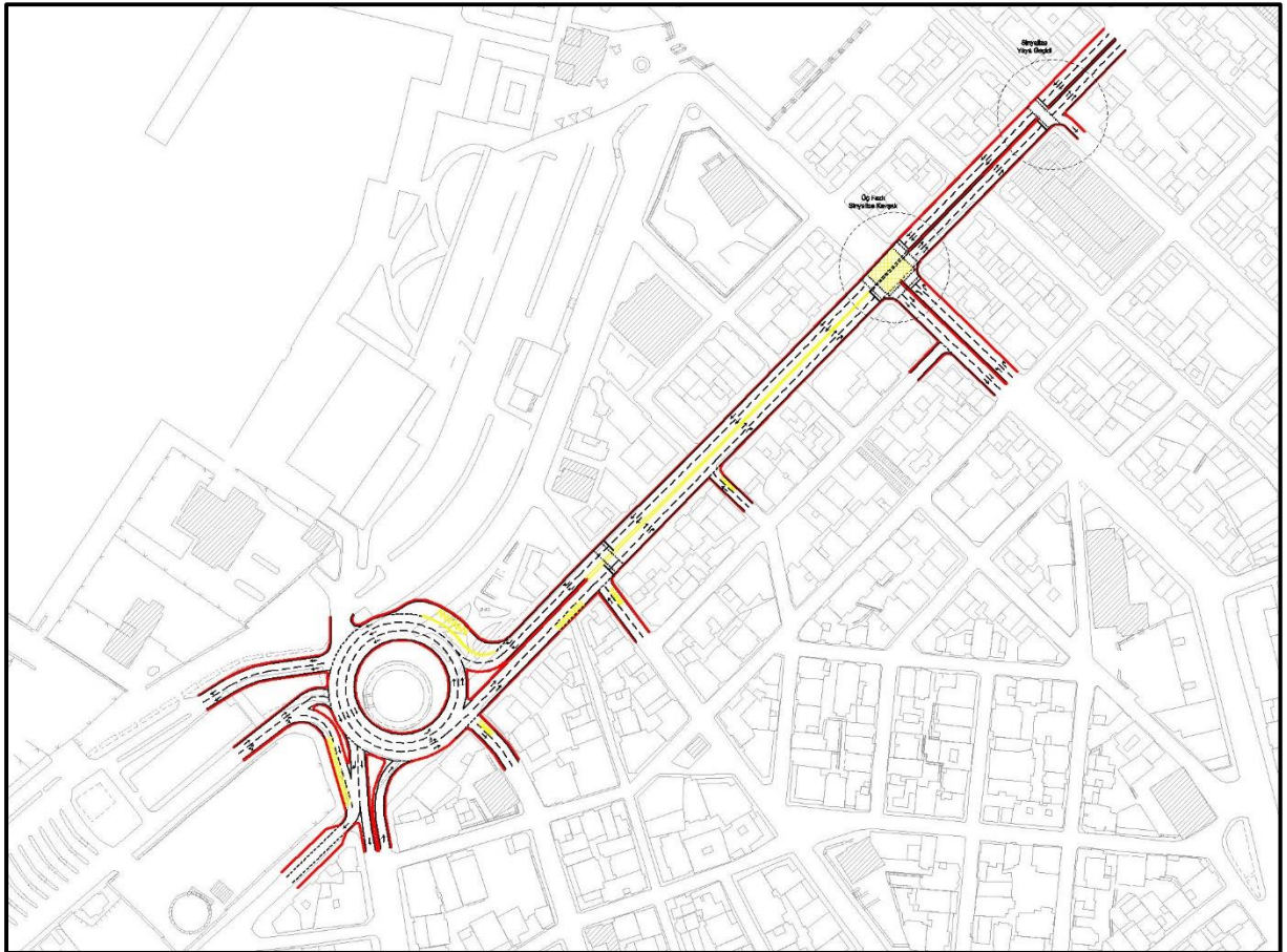
Şekil 5.2 : 1, 2 ve 3 Numaralı Kavşakların Projesi (Alternatif-2)
