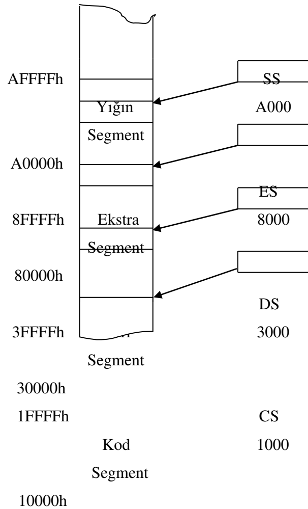
Şekil.2.4. Segment saklayıcıları ile adreslenen bir hafıza haritası
