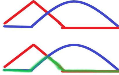
Şekil 7: Üyelik fonksiyonlarının kesişimi
