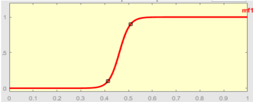
Şekil 48: Sigmoid üyelik fonksiyonu
