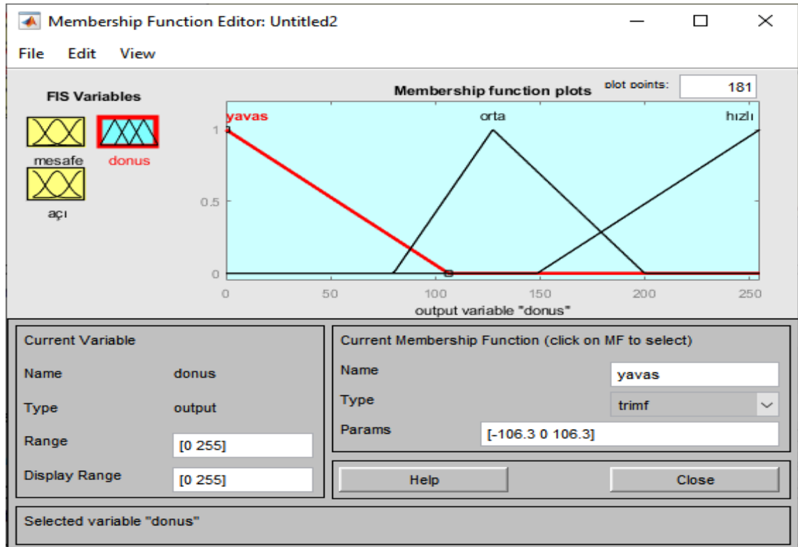
Şekil 62: Üyelik fonksiyonlarının eklenmesinin üçüncüsü
